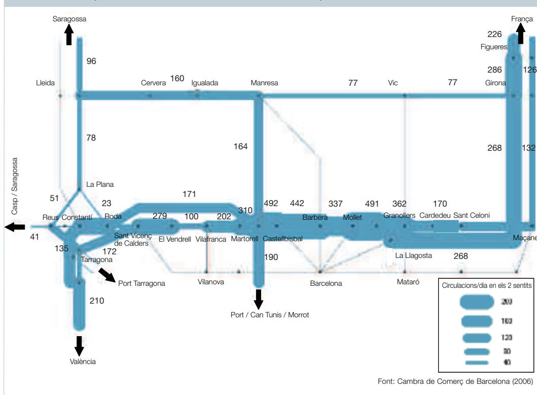
Circulacions totals previstes en l'horitzó 2030 a les línies amb trànsit de mercaderies (amb l'eix transversal ferroviari en servei)
