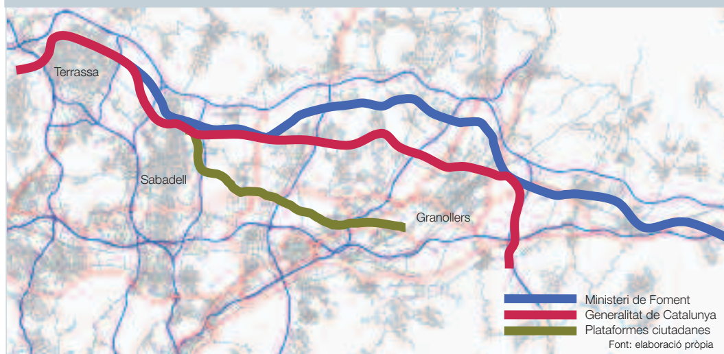
Alternatives de traçat plantejades per a la via orbital de Barcelona B-40
